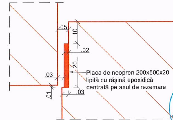
Detaliul "A" Sc. 1:10
